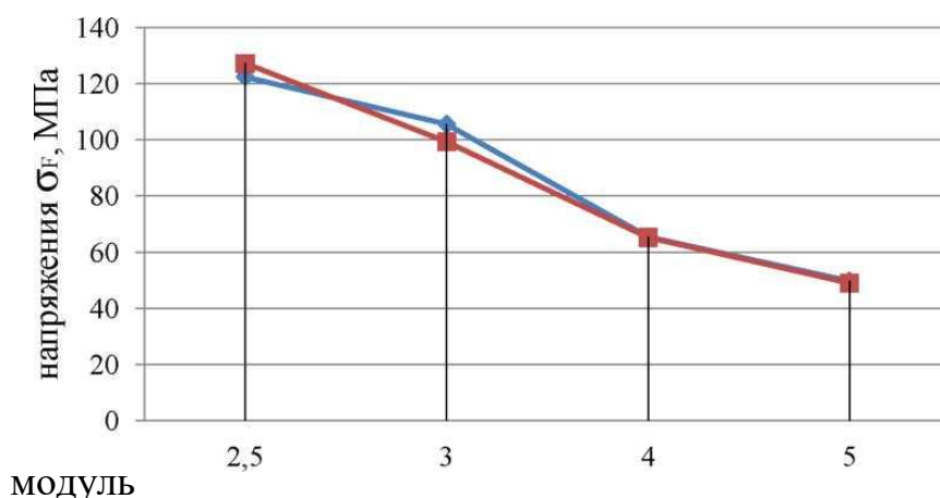
Рисунок 2. Зависимость изгибных напряжений шестерни и колеса от величины модуля.
