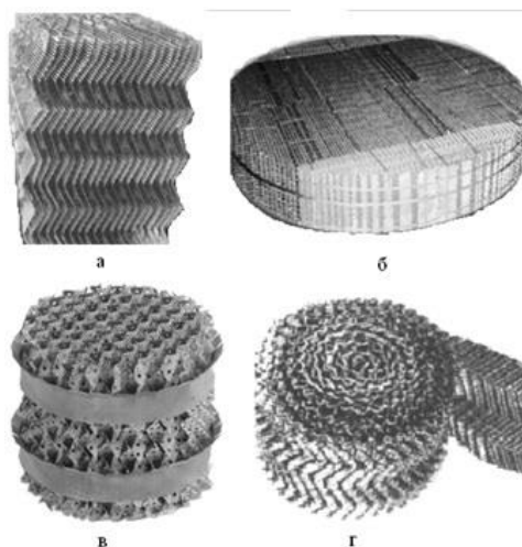
Рисунок 1 - Регулярные насадки: а – Вакупак; б – «Кедр»; в – Меллапак 250; г – насадка Гудлоу
