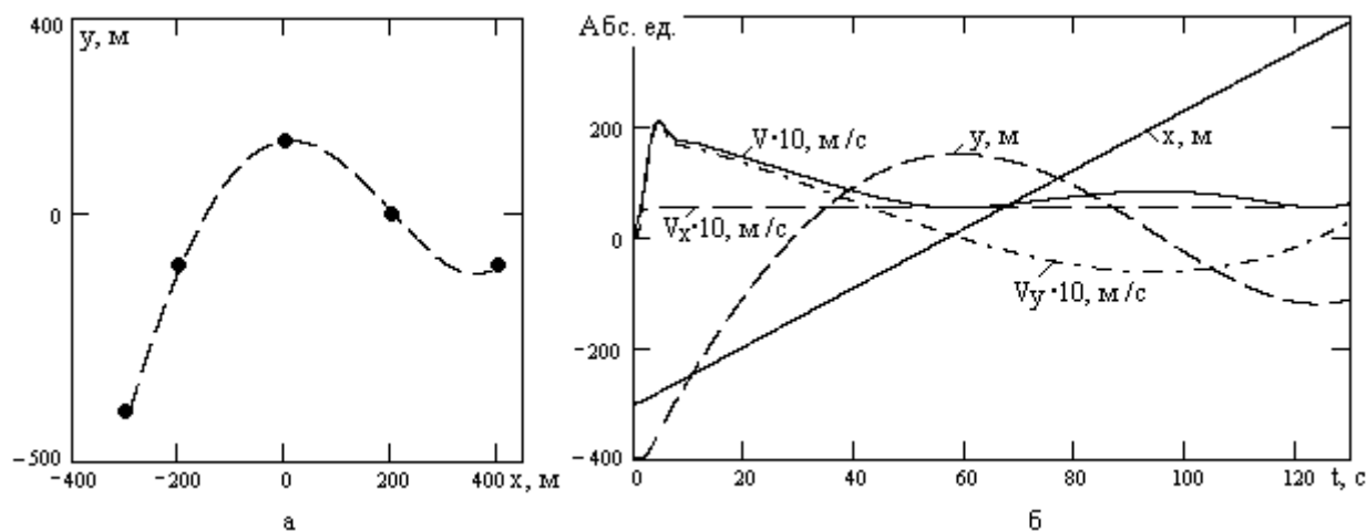
Рисунок 4 – Движение по заданной траектории
