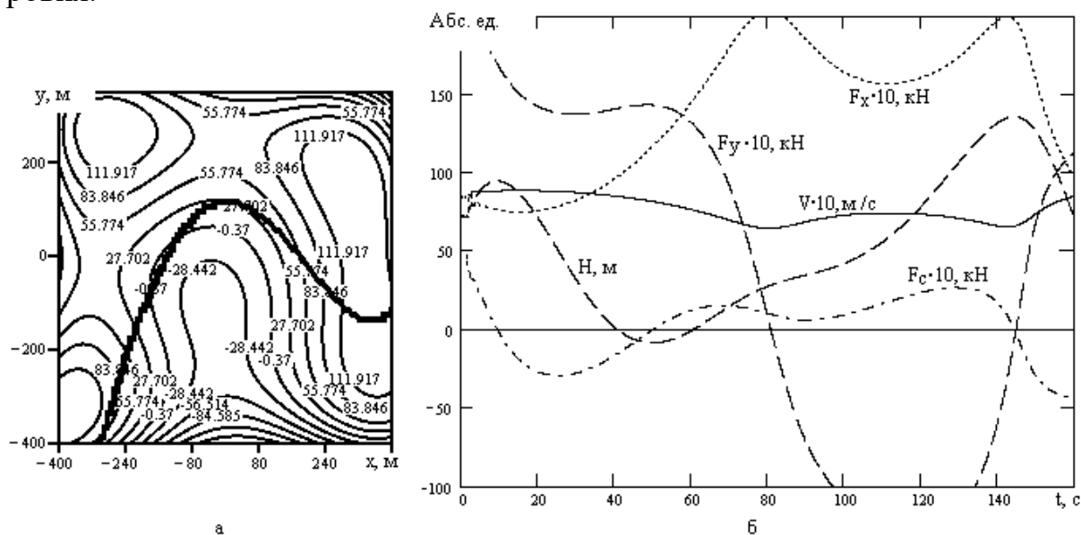
Рисунок 8 – Движение по холмистой поверхности
