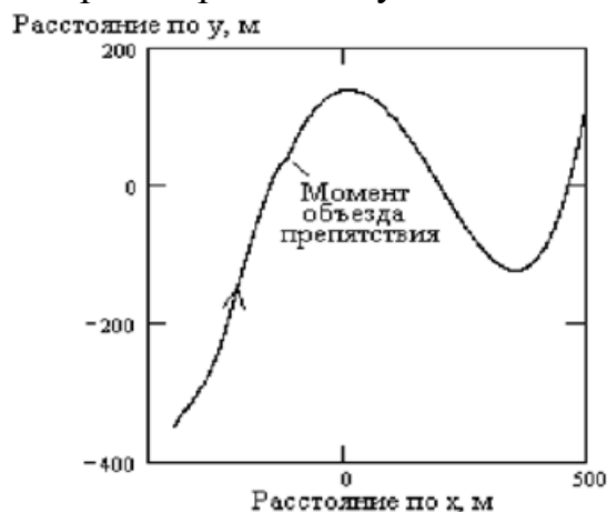
Рис 9а. Общий вид траектории при объезде препятствий
