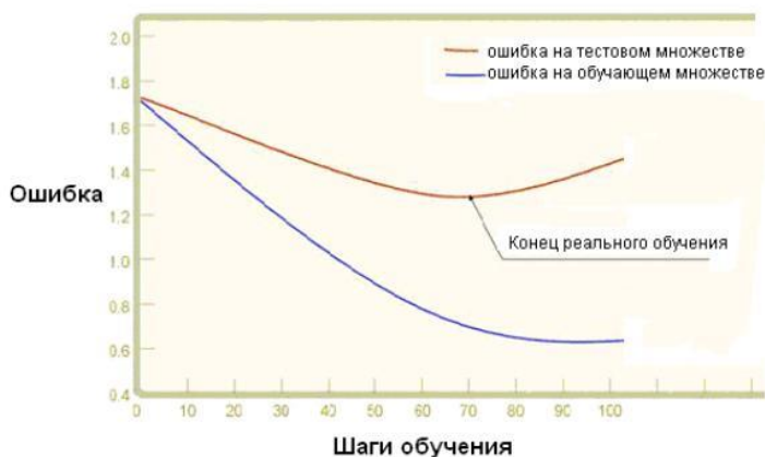
Рисунок 6 - Процесс обучений сети
