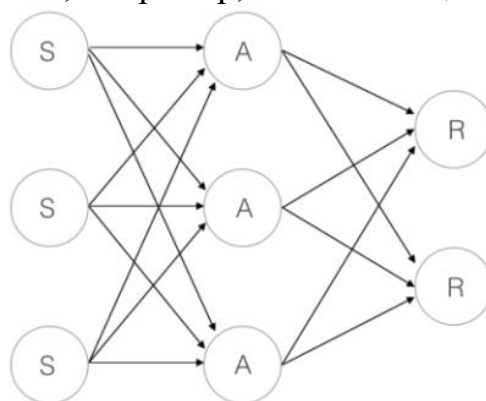
Рисунок 2 - Архитектура персептрона
