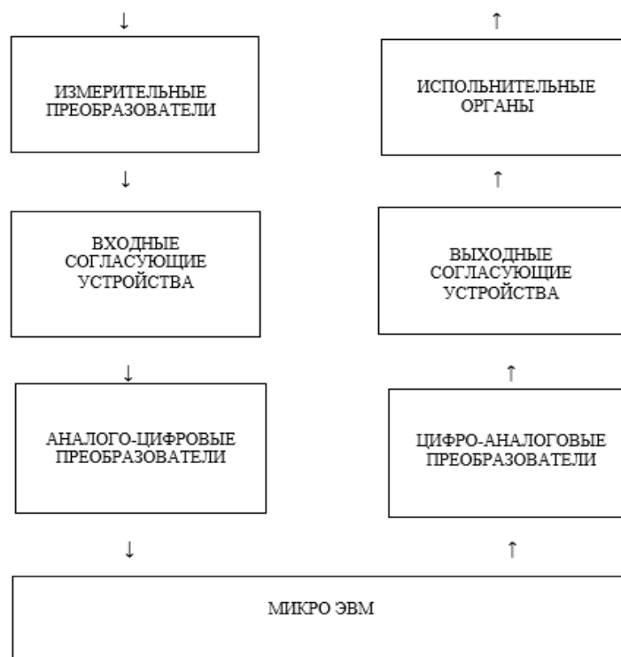
Рис.1. Структурная схема программной защиты
